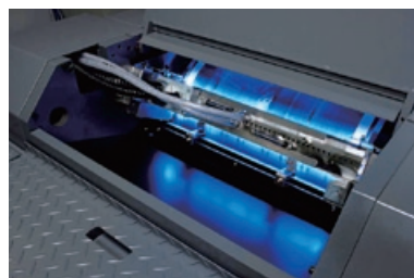
LEDを採用したUV乾燥装置
